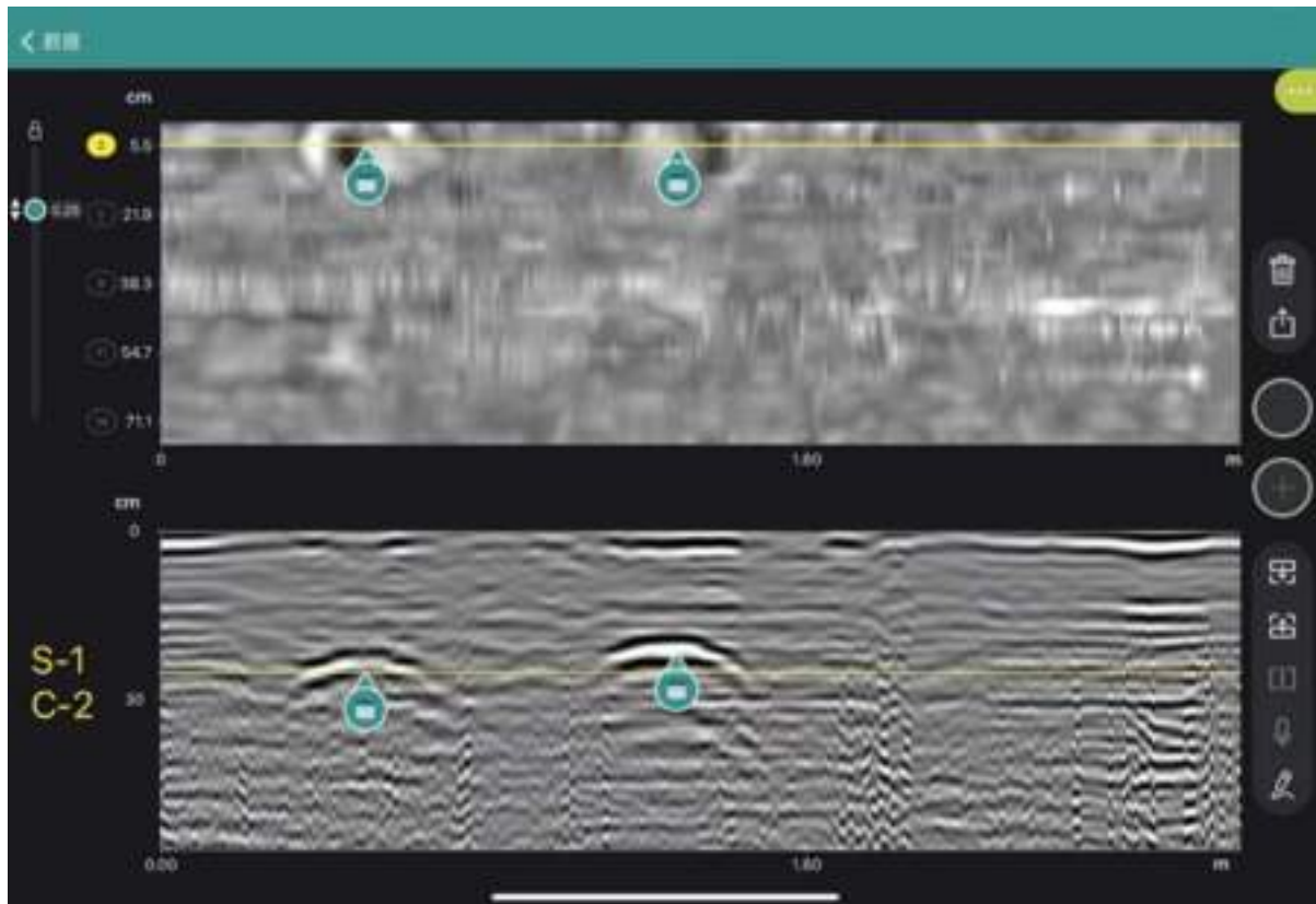
蚁窝的雷达三维图像切片视图（上半部分）和雷达线扫标记（下半部分）
